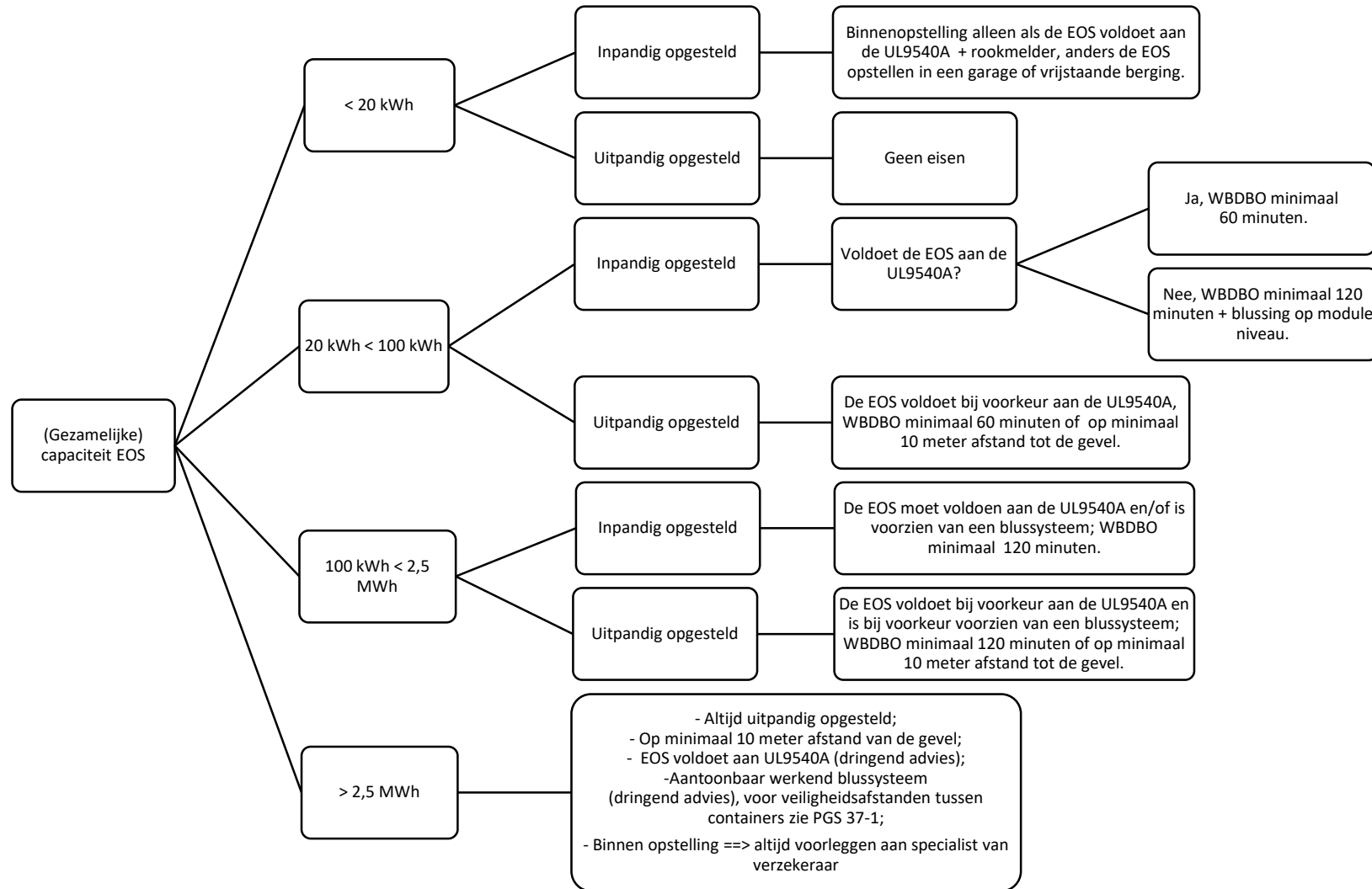
Figuur 1: Blokschema Energieopslagsystemen (EOS) met lithiumhoudende energiedrager (BvT visie)
